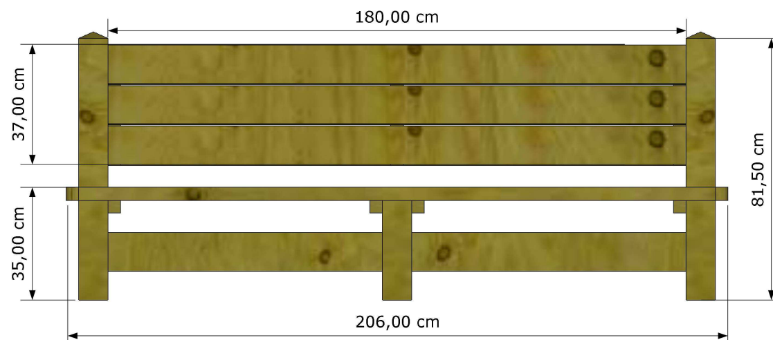
Panchina-V180 – cm. 59x206
