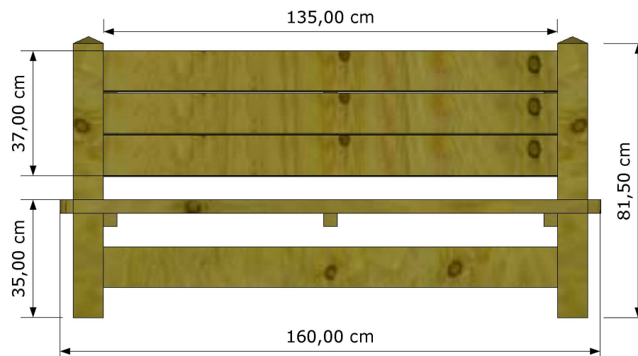
Panchina-V135 – cm. 59x160
